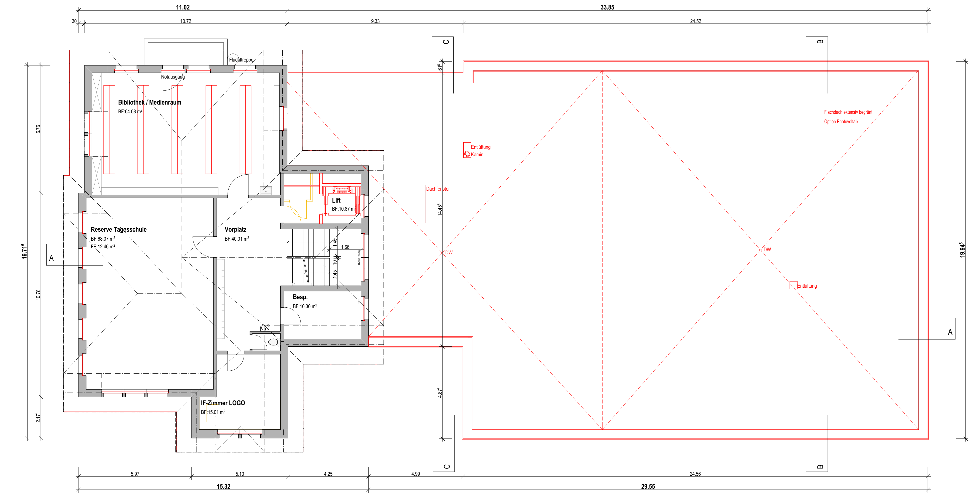
2. obergeschoss
