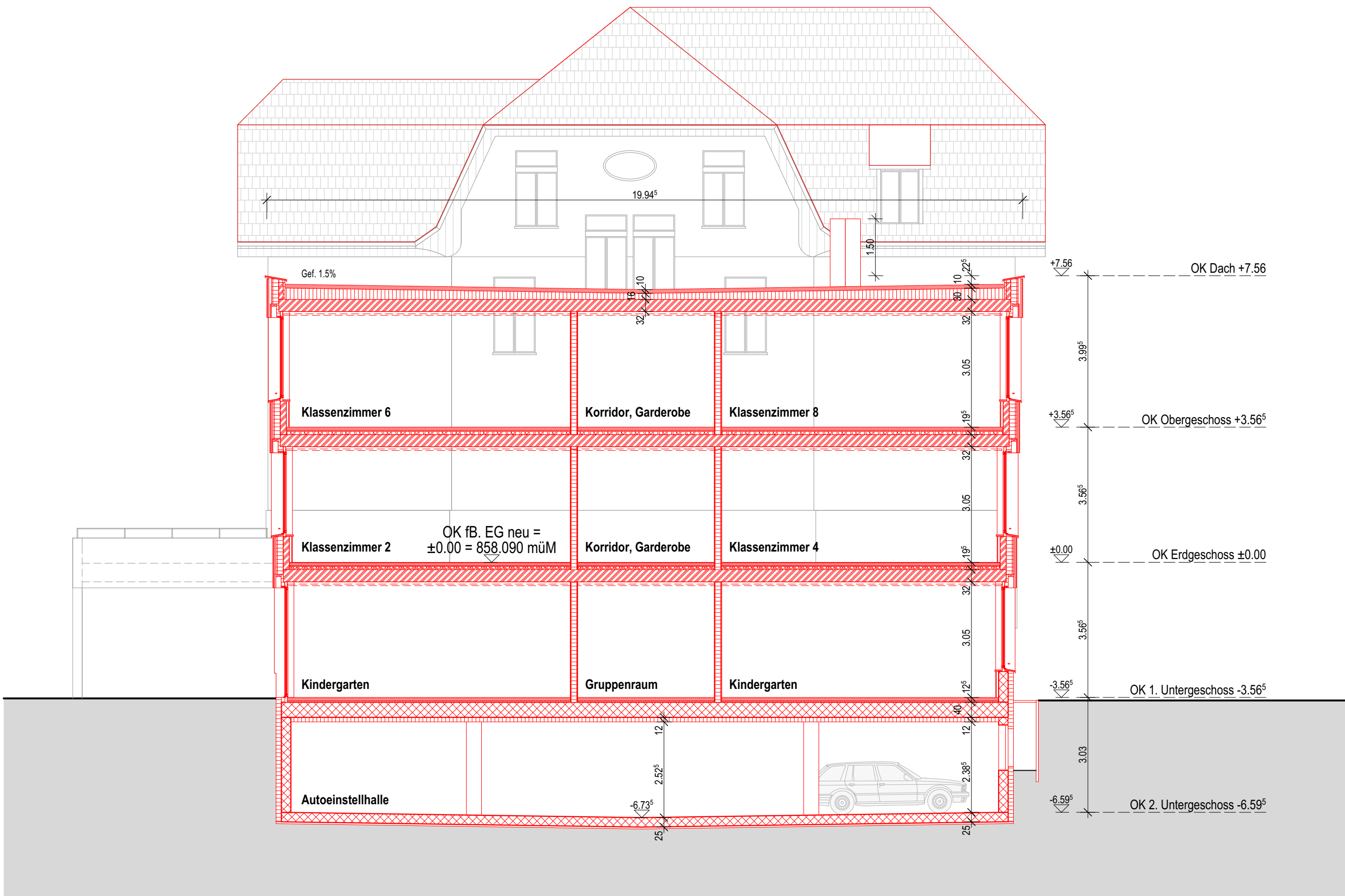
schnitt b-b
