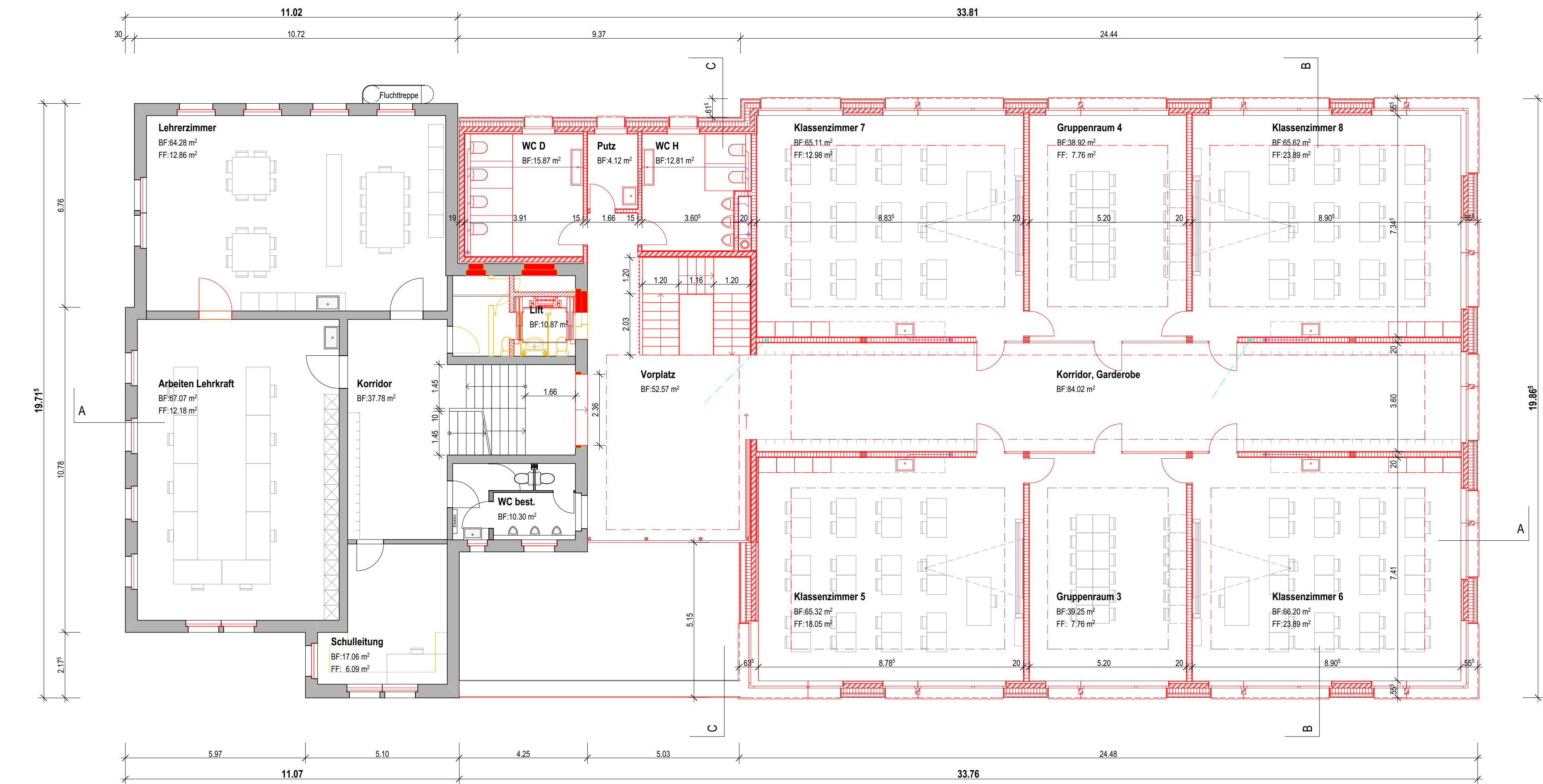
1. obergeschoss
