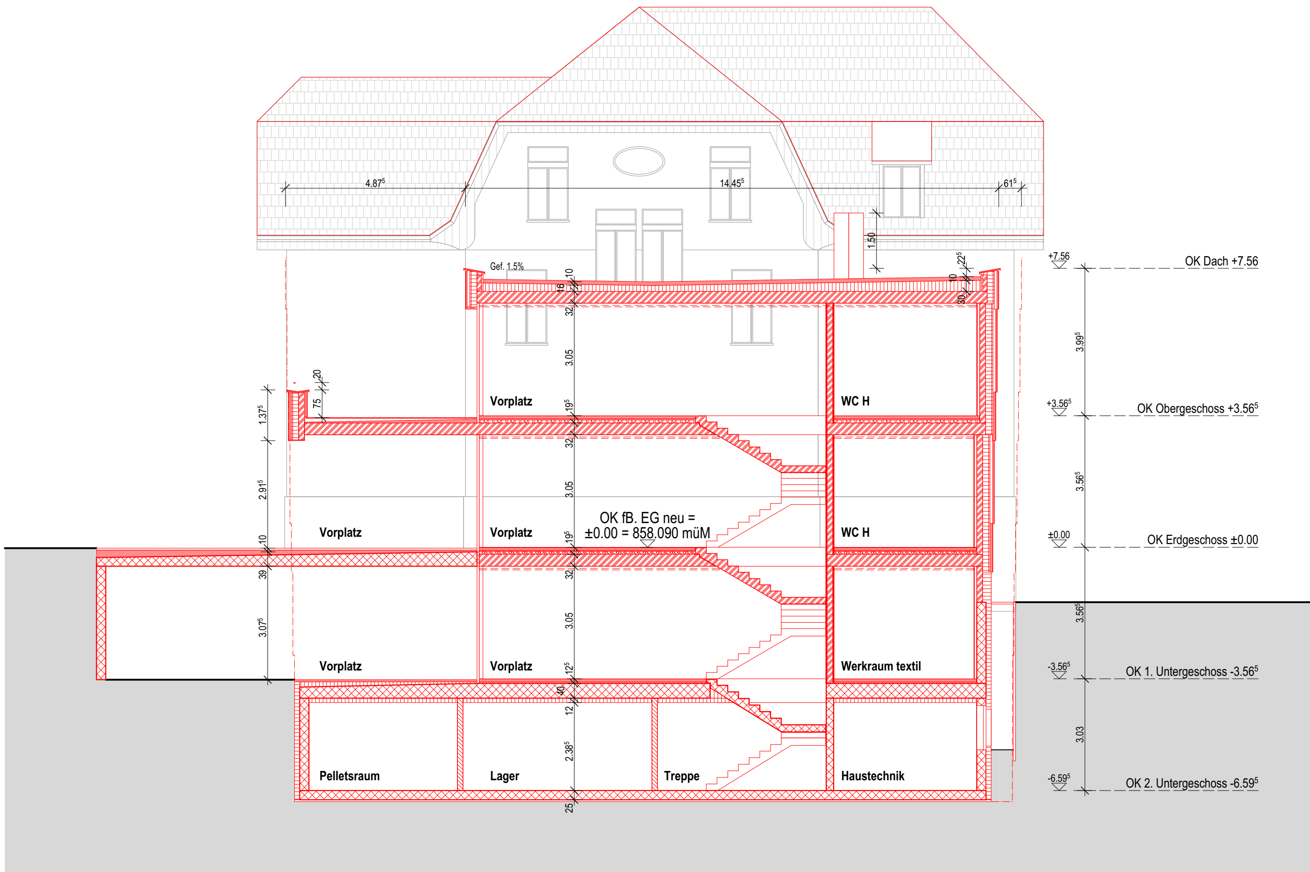
schnitt c-c
