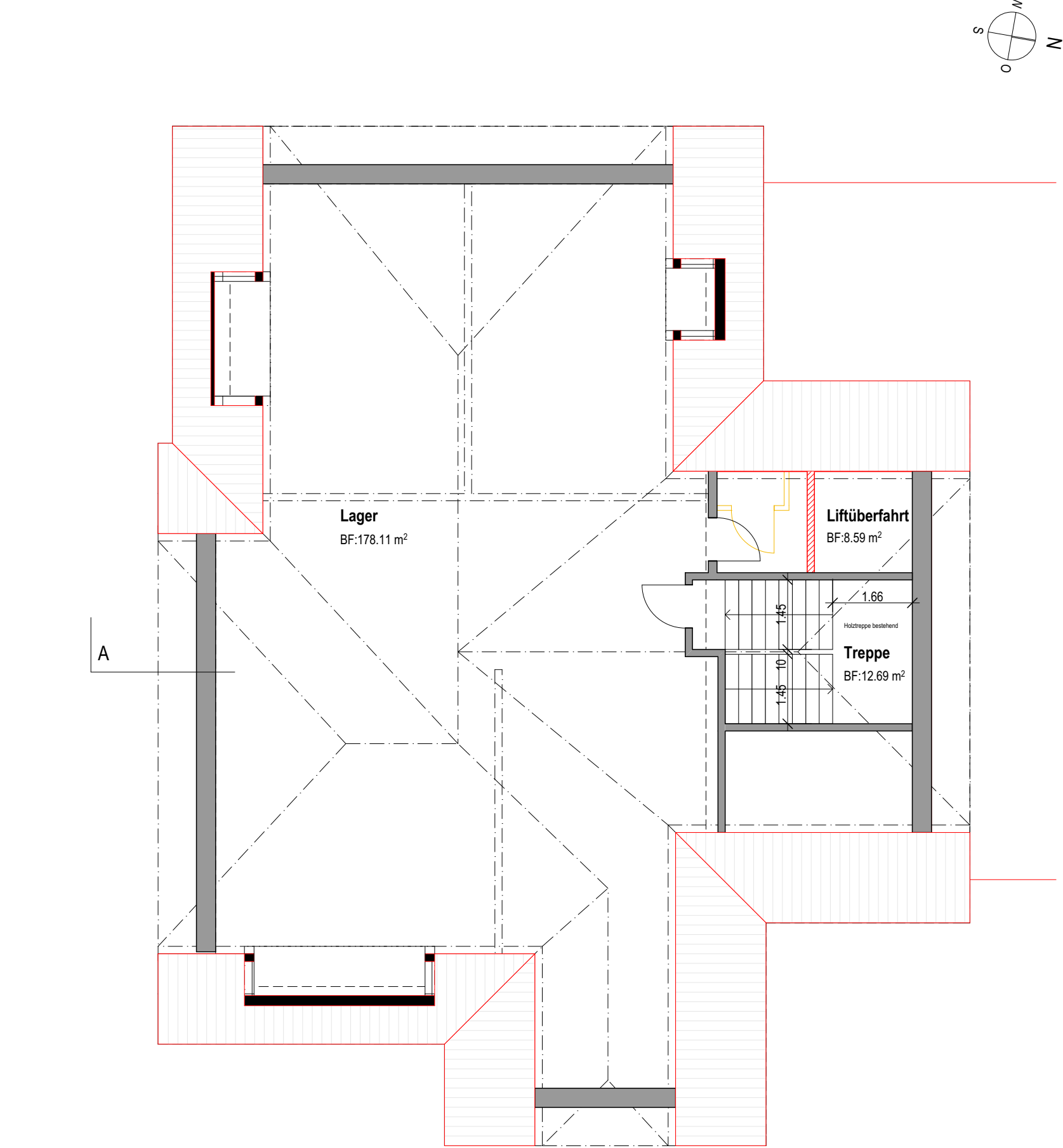
dachgeschoss
